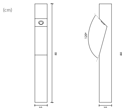
LUMINÁRIA ORQUÍDEA REF. 2555 | LUMINAIRE MODÈLE ORCHIDÉE | ORCHID LAMP
