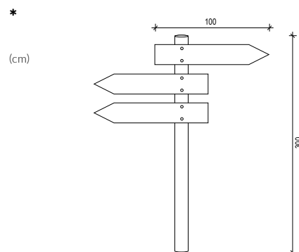
SINALIZAÇÃO SIMPLES REF. 2202 | SIGNALISATION SIMPLE | BASIC SIGNPOST
