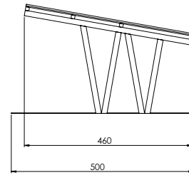
VISTA LATERAL VUE LATÉRALE SIDE VIEW
