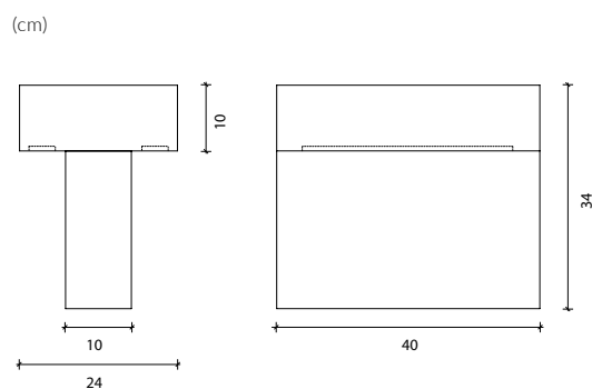
CASOTA DE CÃO PEQUENA REF. 2553 | PETITE NICHE POUR CHIEN | SMALL DOG HOUSE
