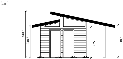
VISTA LATERAL VUE LATÉRALE SIDE VIEW
