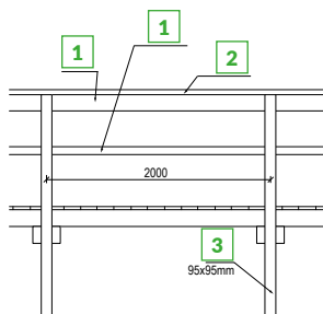
ALÇADO LONGITUDINAL ÉLEVATION LONGITUDINALE LONGITUDINAL ELEVATION
